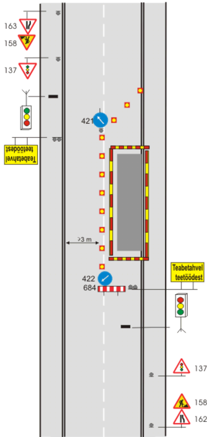
Joonis 20. Ajutiste fooride kasutamine
