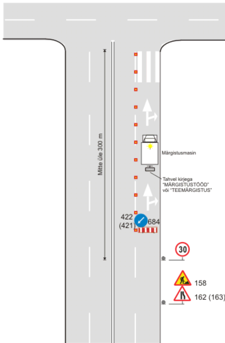
Joonis 31. Eraldussaarte, ülekäiguradade, stoppjoonte, suunanoolte ja muude kirjete märgistamine
