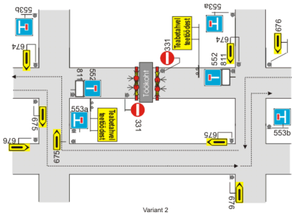
Joonis 35. Liikluse sulgemine tänaval
