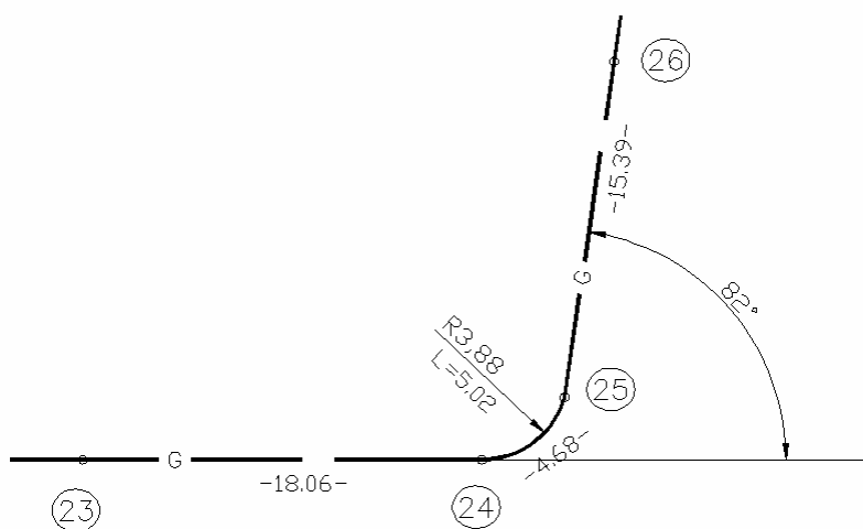
Joonis 2. Gaasitorustiku painutatud käänaku kujutamine.
