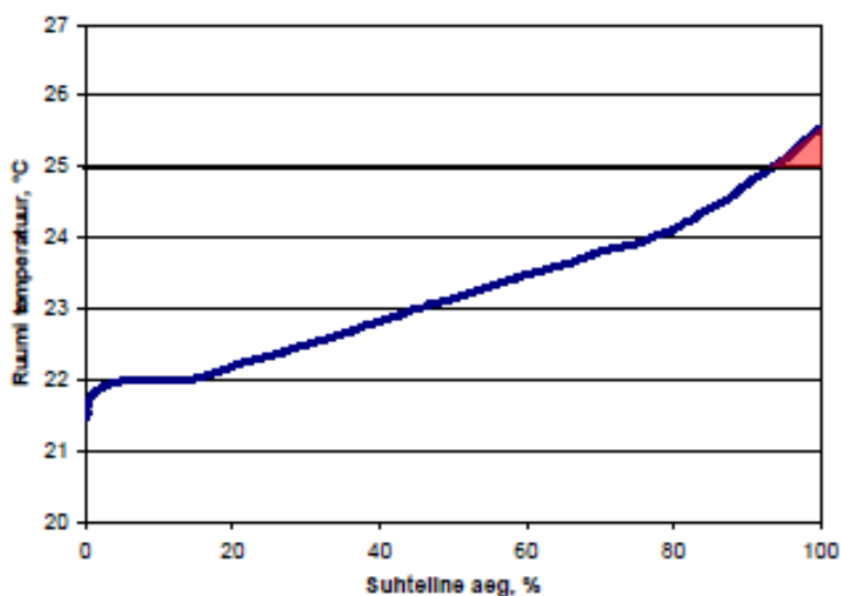
Ruumitemperatuuri kestuskõver
