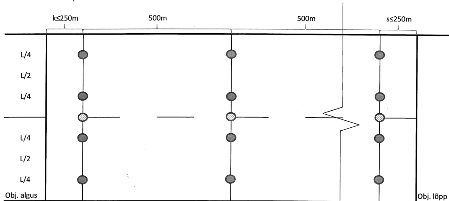
Joonis 1 Kattest puurkehade võtmise skeem
