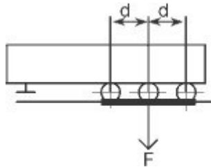
Joonis 49. Kolmeteljelisele telikule mõjuv koormus ( F ) ja telgede vahekaugused ( d )
