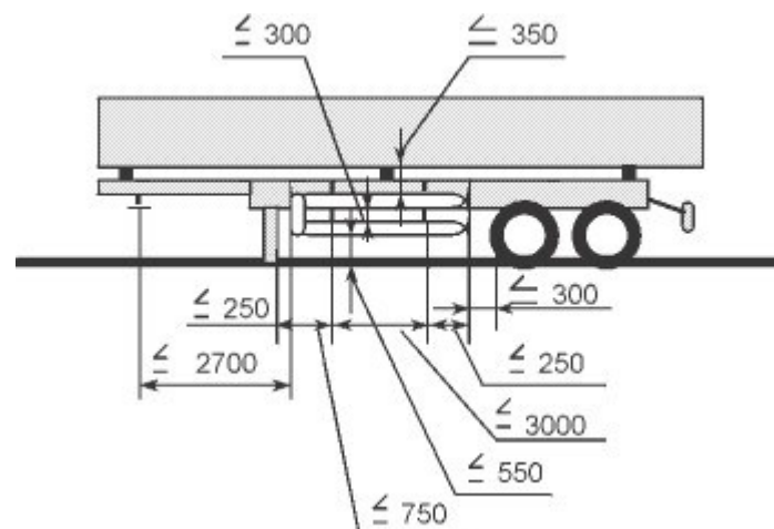
Joonis 21. Külgmise allasõidutõkke asukoht täishaagisel
