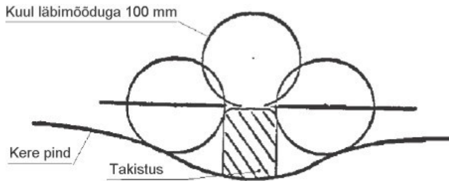
Joonis 14. Ø 100 mm kuuli veeretamine üle kere pinnal olevast takistusest
