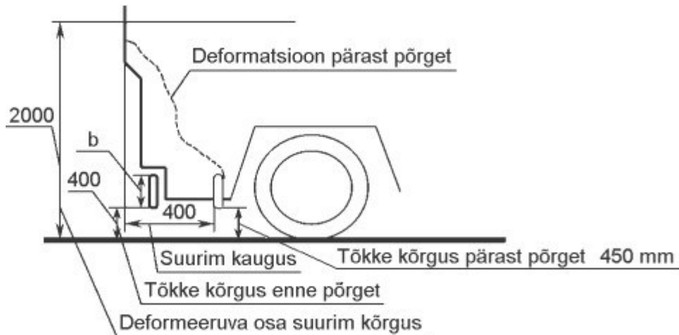
Joonis 19. Tõkke külgsaates. Lubatud deformatsioonid. b – tõkke profiili laius
