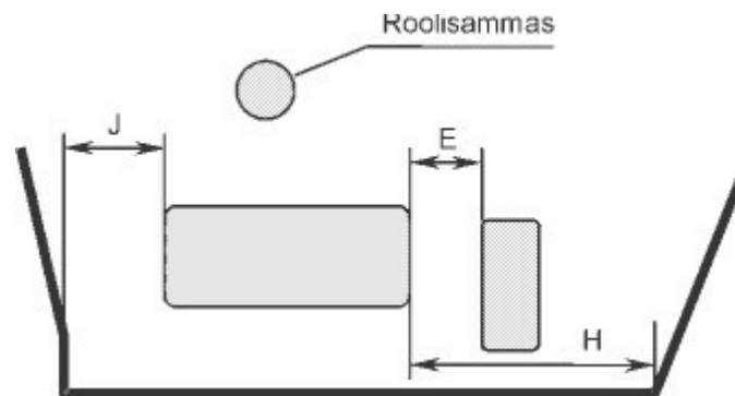
B. Kahe pedaali asend. Mõõtmed on toodud tabelis 7 Joonis 15. Pedaalide asendid
