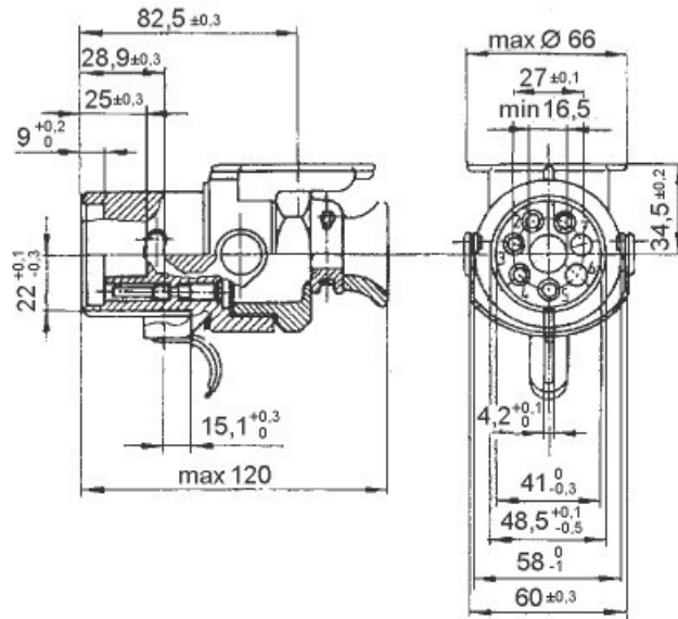
Joonis 36. ABS pidurisüsteemi pistik
