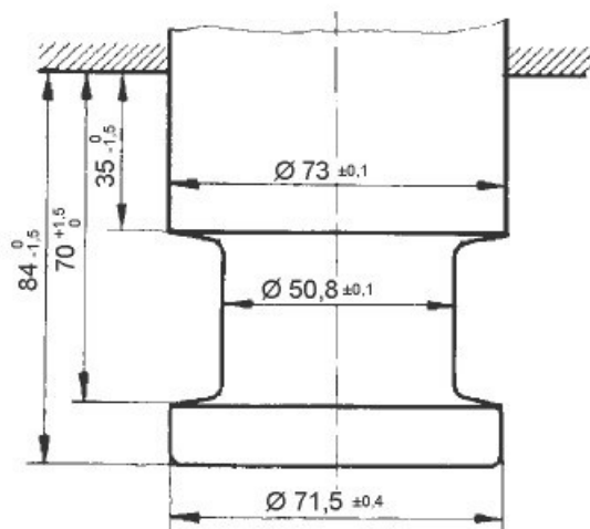
Joonis 23. Poolhaagise veopolt « \varnothing 50 » mm
