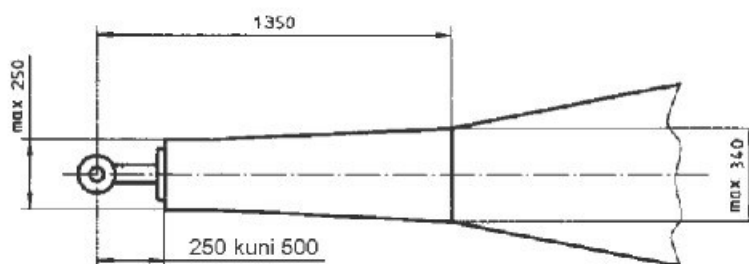
Joonis 29. Kesktelghaagise tiisli esiosa
