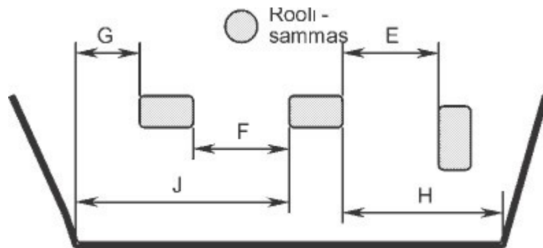
A. Kolme pedaali asend. Mõõtmed on toodud tabelis 6
