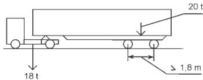
Joonis 47. Autorongi koormus ja poolhaagise tandemtelgede asetused
