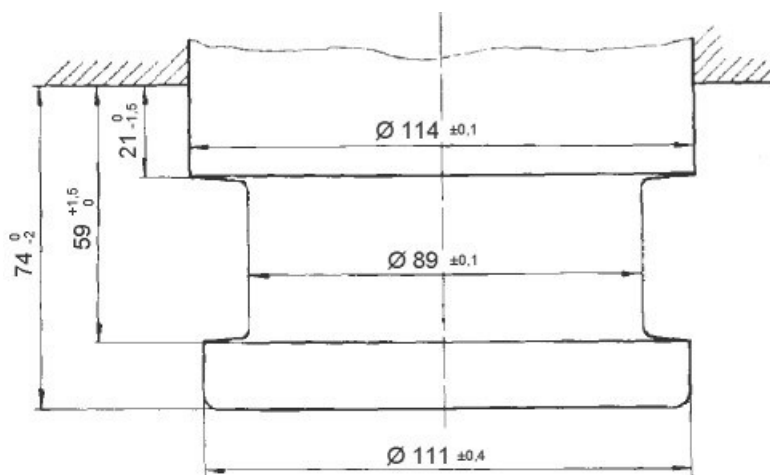
Joonis 24. Poolhaagise veopolt «Ø 90» mm
