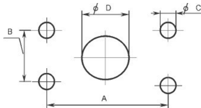
Joonis 26. Haakeseadme kinnituspoldide avad
