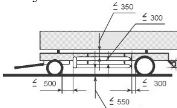
Joonis 20. Külgmise allasõidutõkke asukoht mootorsõidukil
