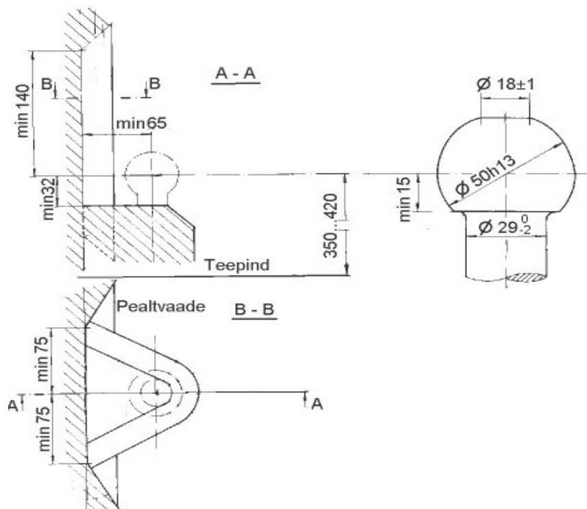
Joonis 27. Haakeseadme kuulpolt ja selle paigaldamise mõõtmed
