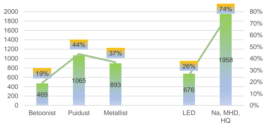
Joonis 9. Valgustid ja mastid Saku vallas (allikas: Saku Vallavalitsus)
