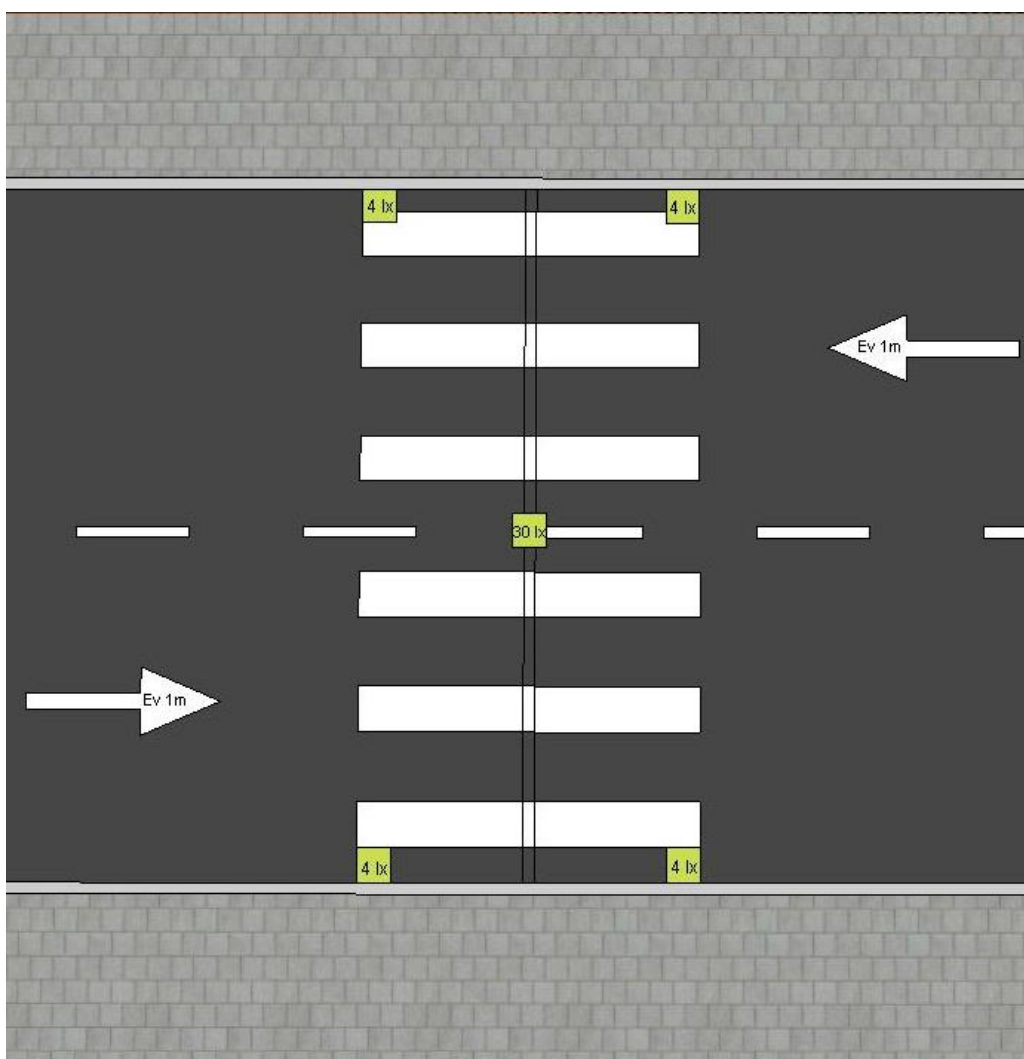
Skeem 4 Ülekäiguraja valgustiheduse mõõtmine
